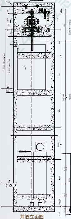
井道立面图
